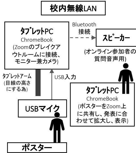
図3 配信用端末セットの配線図
